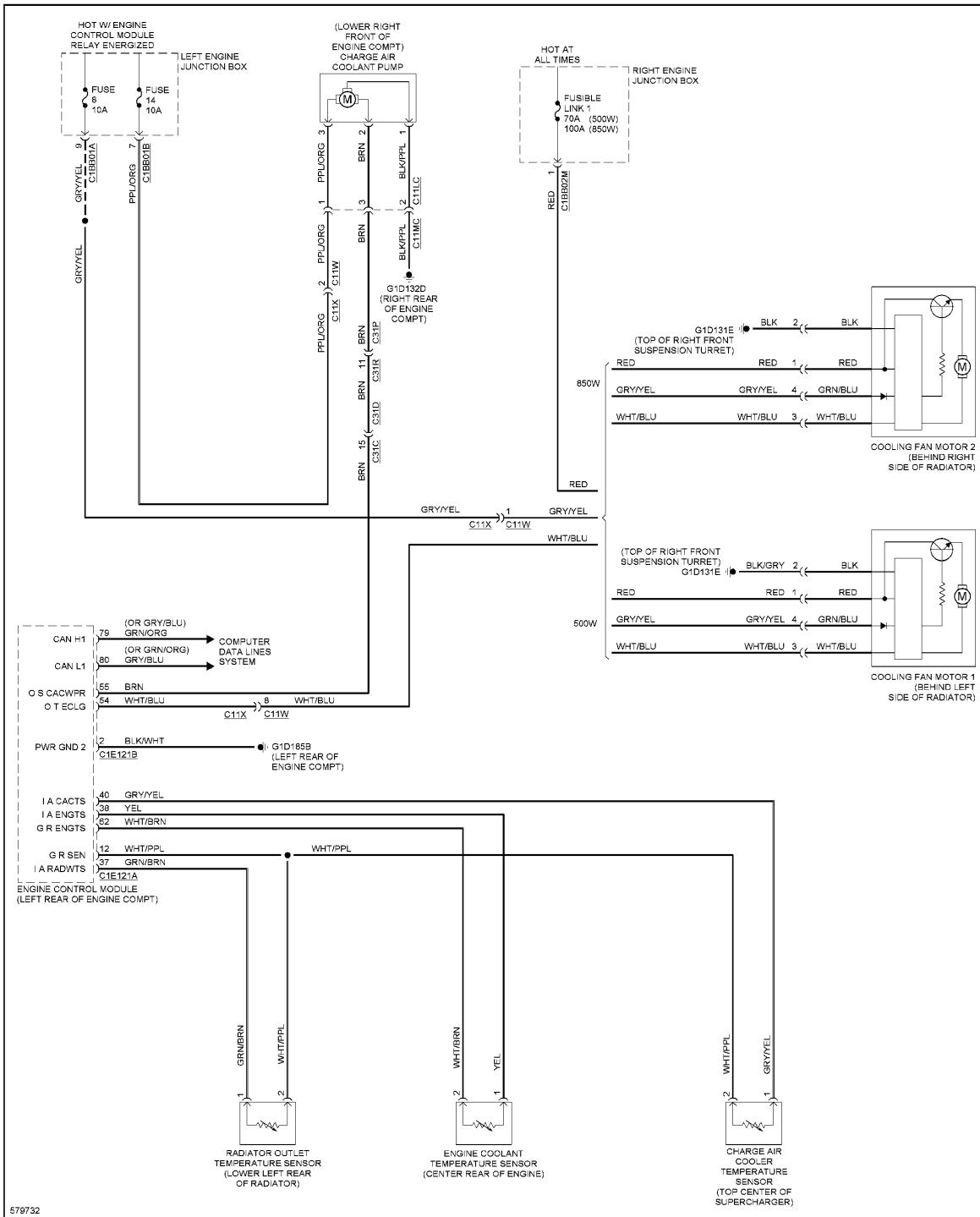
Fig. 15: Cooling Fan Circuit
