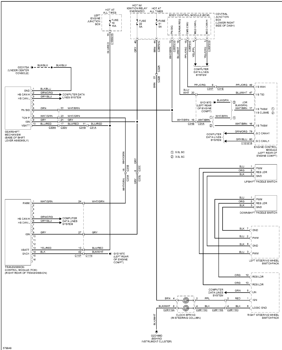
Fig. 131: A/T Circuit
